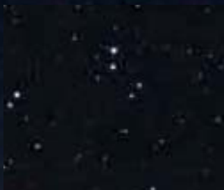
すばる望遠鏡がとらえたくじら座の方向の深宇宙領域。
