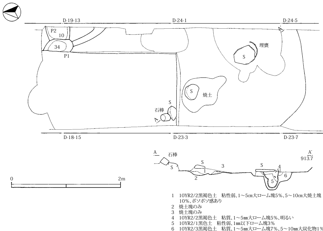
第 8 図 第 105 号住居址 (1/40)
