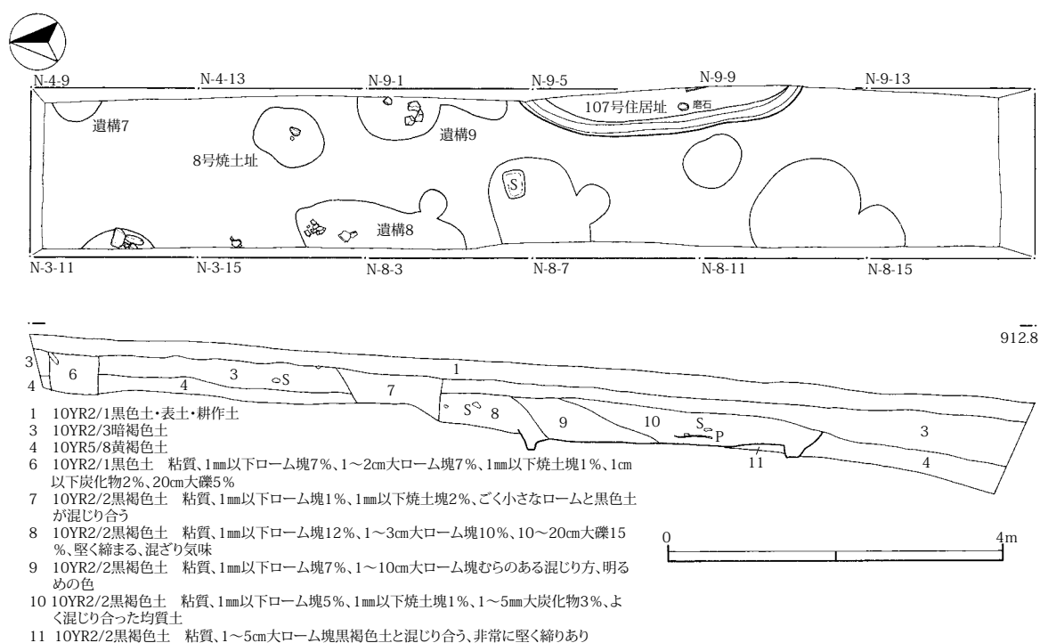
第 11 図 南北トレンチ平面・断面図 (3)(1/80)
