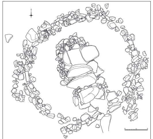
永明寺山古墳 平面図
