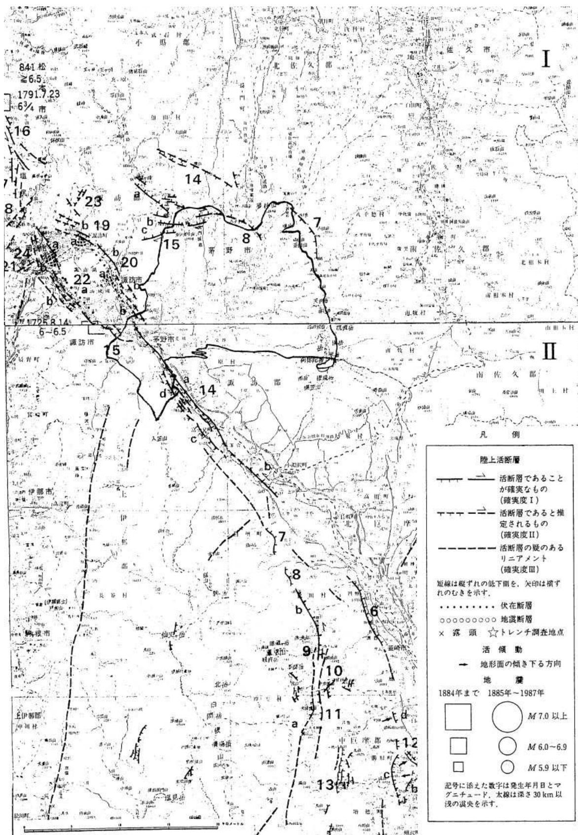
茅野市周辺における活断層の分布状況
