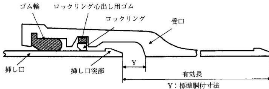
図 3-4-2 NS形ダクタイト鋳鉄直管の継手構造
