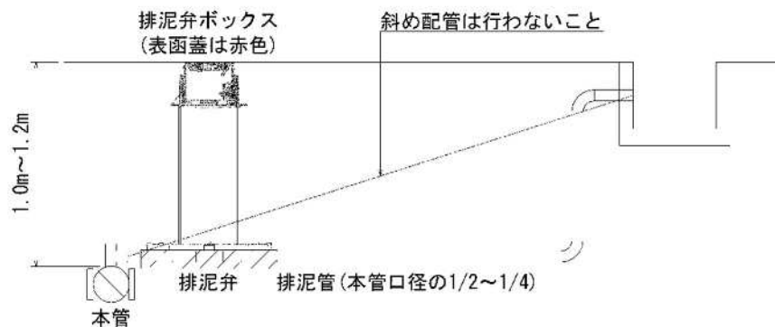
図 3-12-6 泥吐（排泥）管工の標準図
