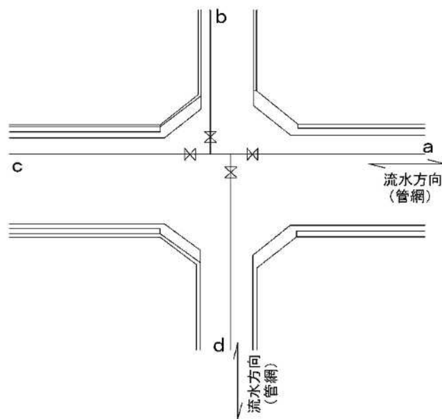
図 3-12-2 仕切弁設置図 (2)
