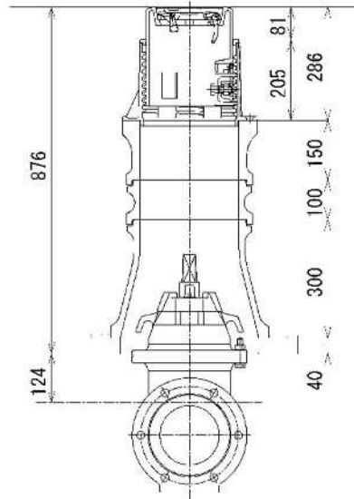
図 3-12-4 仕切弁筐標準図 (例: \phi 150 \text{ mm} \cdot \text{DP}=1.0\text{m} の場合)
