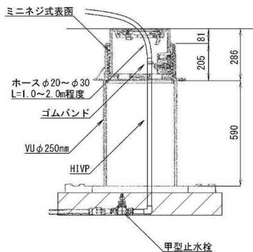
図 3-12-7 地下式排泥構造図
