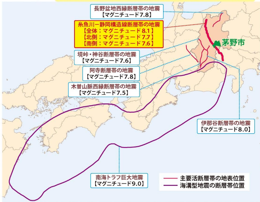
長野県周辺の主要な活断層の分布と想定される地震規模
