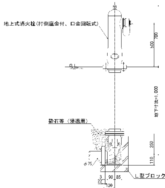
図 3-1-1-2-5 地上式消火栓の設置図
