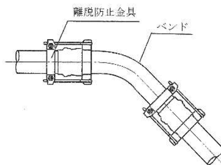
図 3-6-4 離脱防止金具の装着
