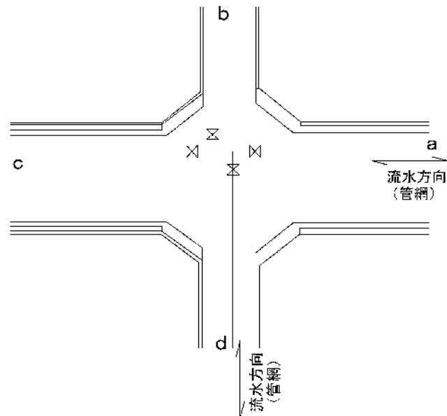
図 3 - 1 1 2 - 2 仕切弁設置図 (2)
