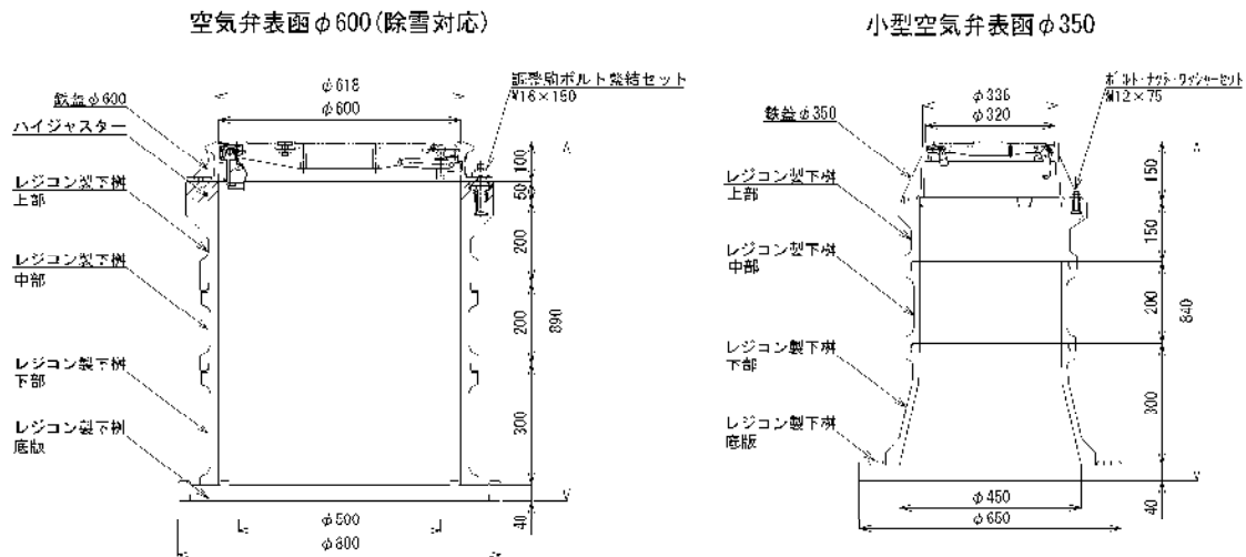
図3-1-12-8 空気弁筐標準図（例：本管 DP=1.0m の場合）
