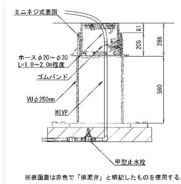
図3-1-12-7 地下式排泥構造図
