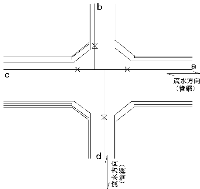
図 3 - 1 1 2 - 3 仕切弁設置図 (3)
